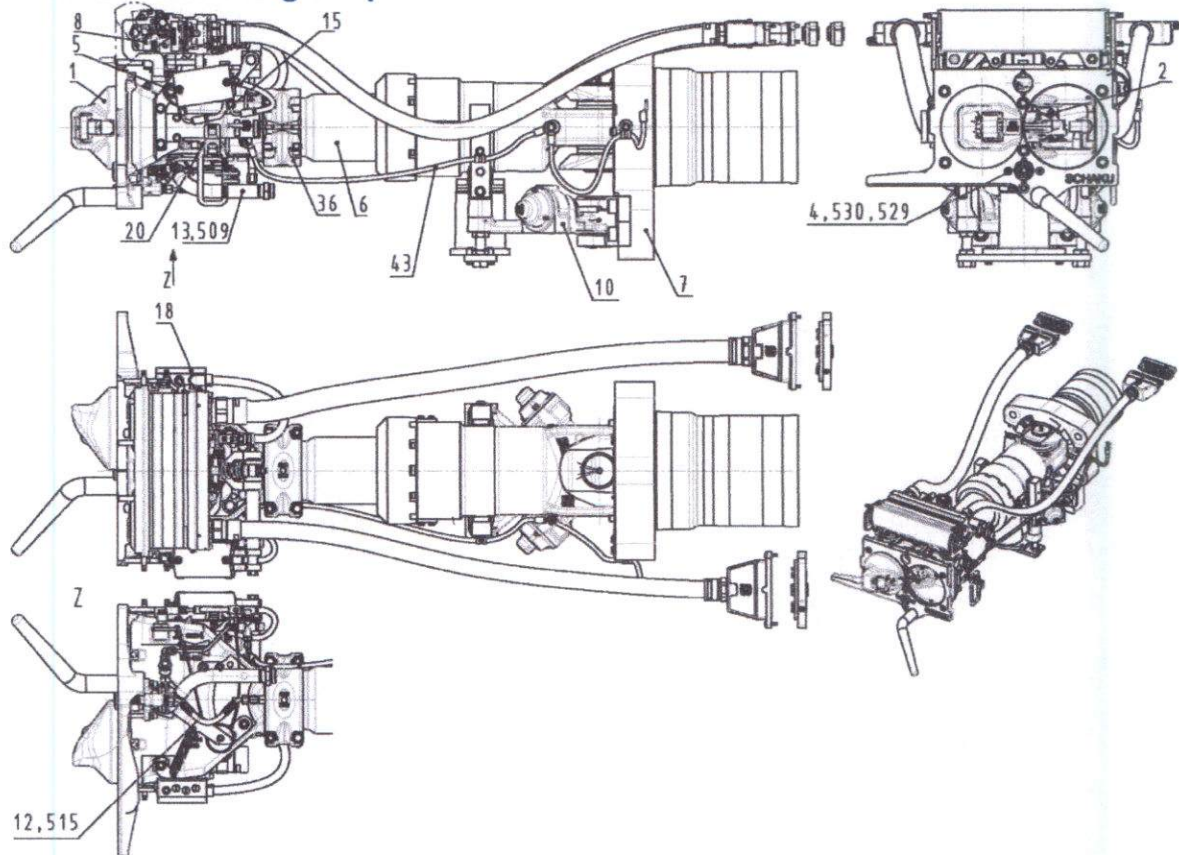
Fig. 134 Scharfenberg coupler 010.775
