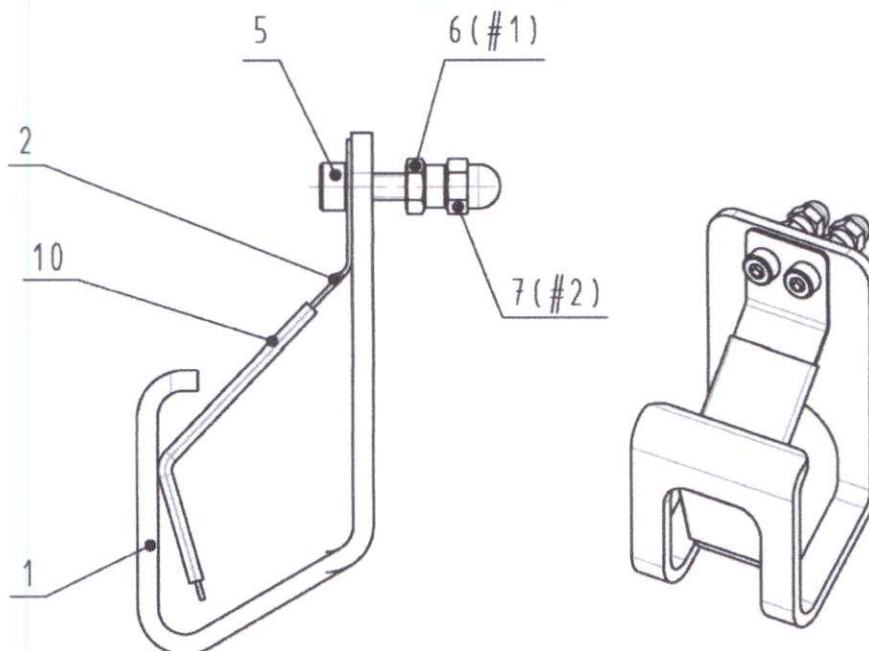
Fig. 159 Handle holder 020.031.01.03 "10.01"
