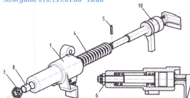
Fig. 138 Stem guide 010.139.01.06 "10.08"
